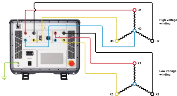
Conexión del TRT500 a un transformador trifásico
