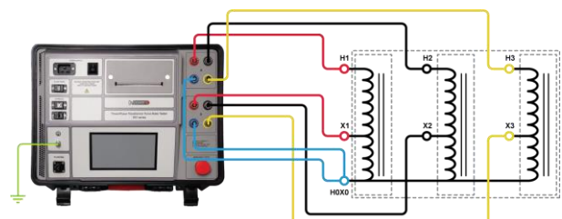
Conexión del TRT400, TRT250, TRT100 a un autotransformador trifásico
