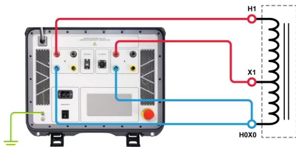
Conexión del TRT500 a un autotransformador monofásico
