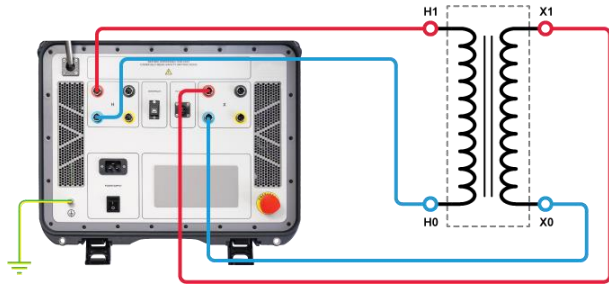
Conexión del TRT500 a un transformador monofásico
