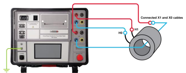
Conexión del TRT400, TRT250, TRT100 a un transformador de corriente amontado
