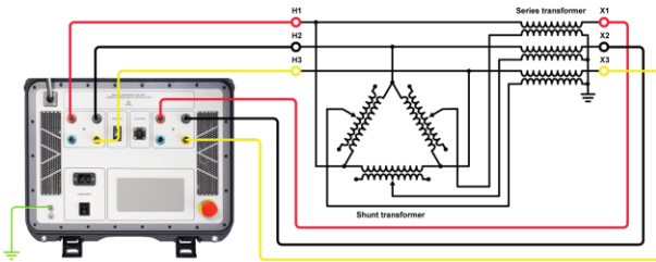
Conexión del TRT500 a un transformador desfasador
