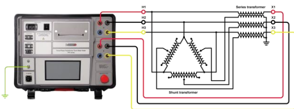
Conexión del TRT400, TRT250, TRT100 a un transformador desfasador
