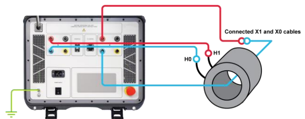
Conexión del TRT500 a un transformador de corriente amontado
