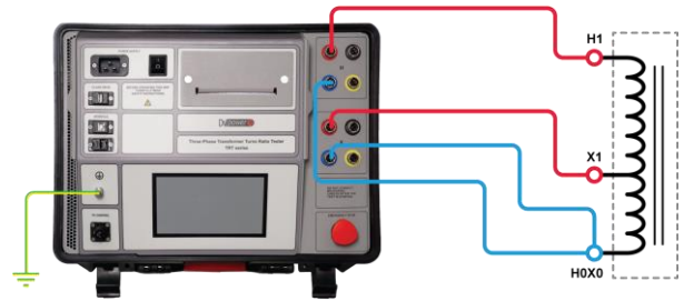
Conexión del TRT400, TRT250, TRT100 a un autotransformador monofásico
